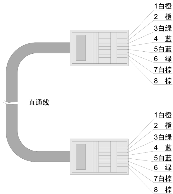
图C-4 直通线两端线序示意图
