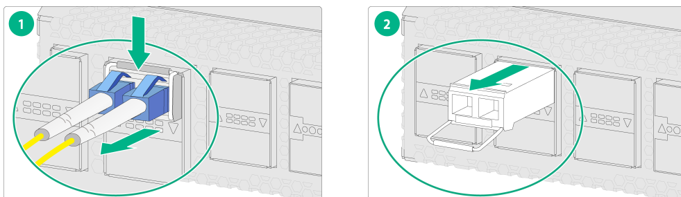
图4-5 拆卸光模块（LC 型接口）
