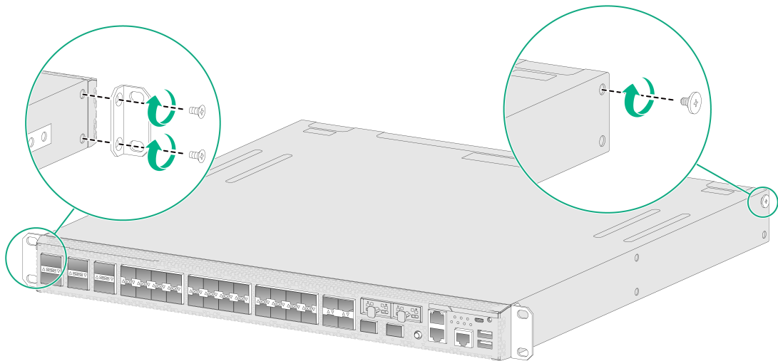
图2-3 安装前挂耳和承重螺钉
