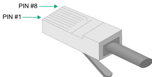
图C-3 RJ-45 连接器引脚序号示意图
