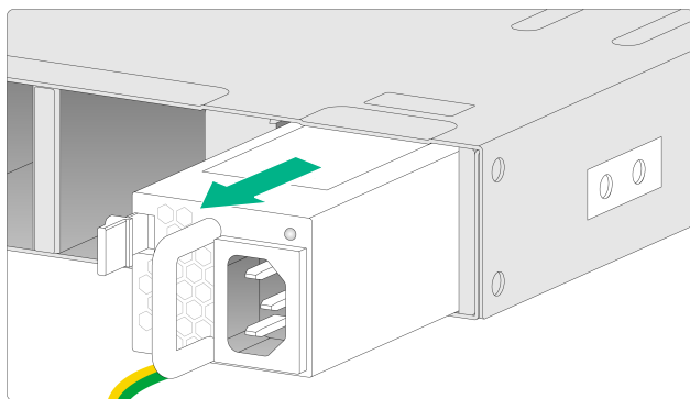
图4-1 拆卸电源模块
