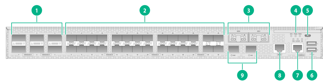
图A-1 设备前视图
