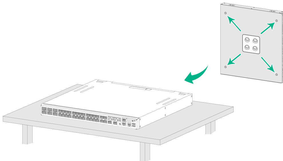
图2-1 工作台安装方式
