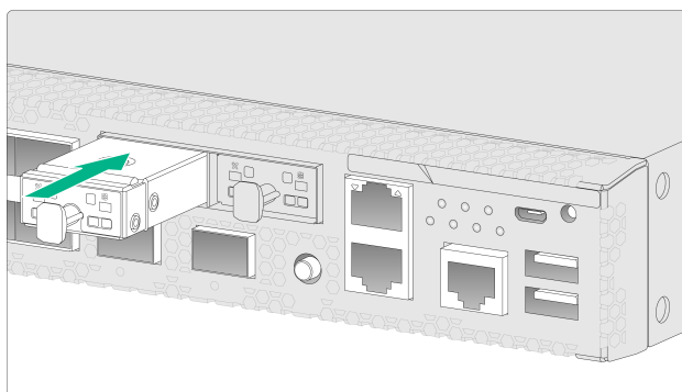
图2-14 安装硬盘
