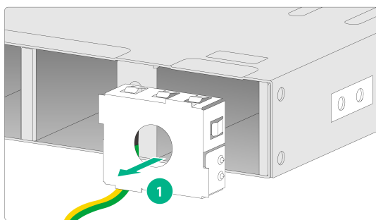
图2-11 拆卸电源假面板
