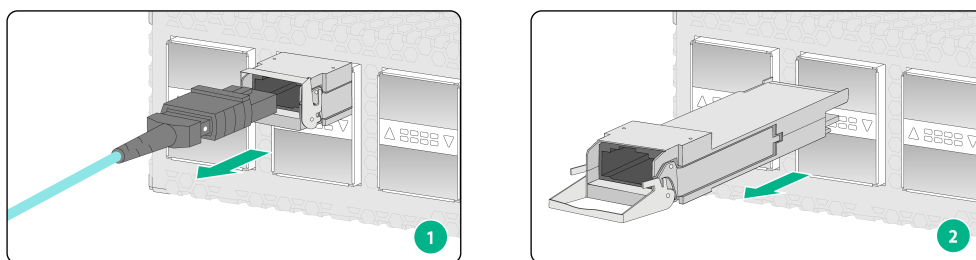
图4-6 拆卸光模块（MPO 型接口）
