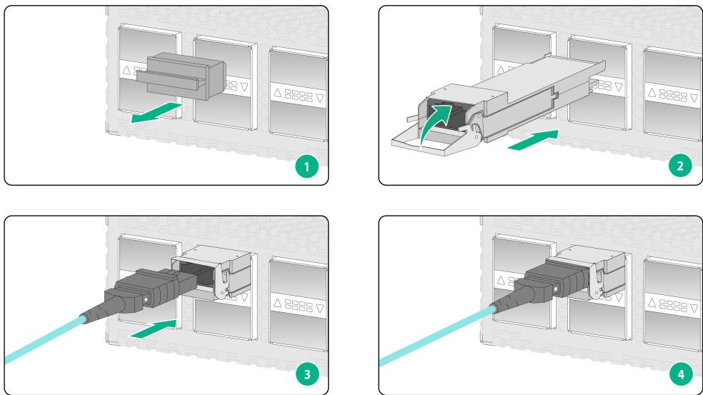
图2-22 安装光模块和光纤示意图（MPO 型接口）
