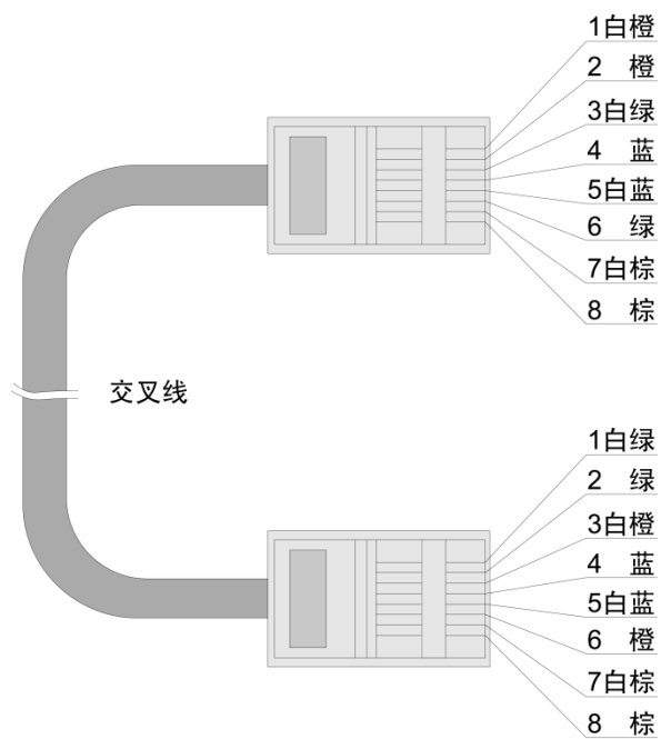
图C-5 交叉线两端线序示意图
