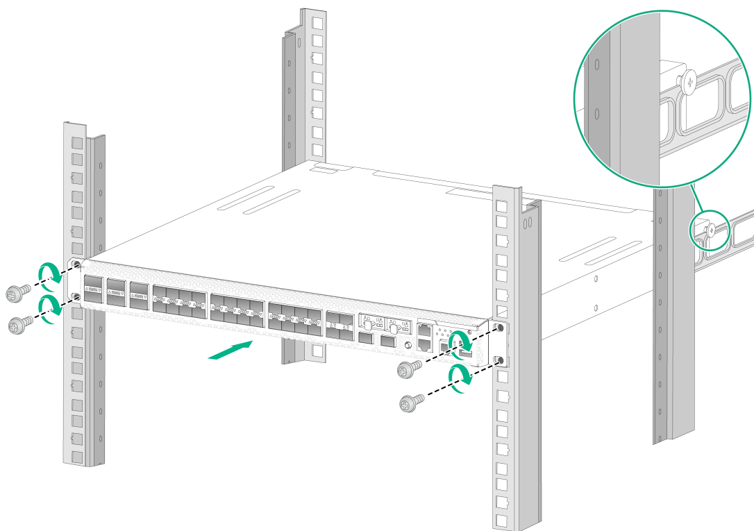
图2-7 安装设备到机柜（后挂耳反装）
