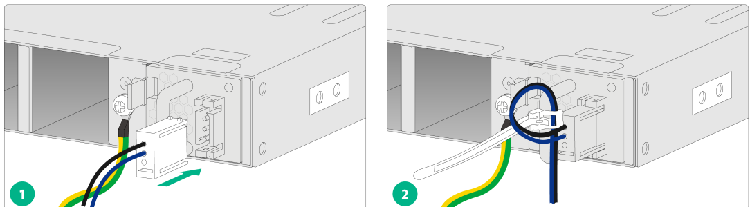
图2-24 连接直流电源线
