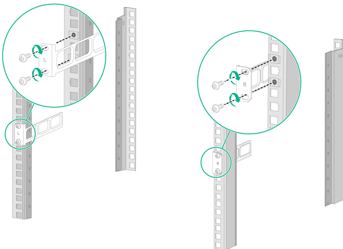
图2-4 安装后挂耳（后挂耳正装）
