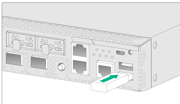
图2-15 安装 U 盘
