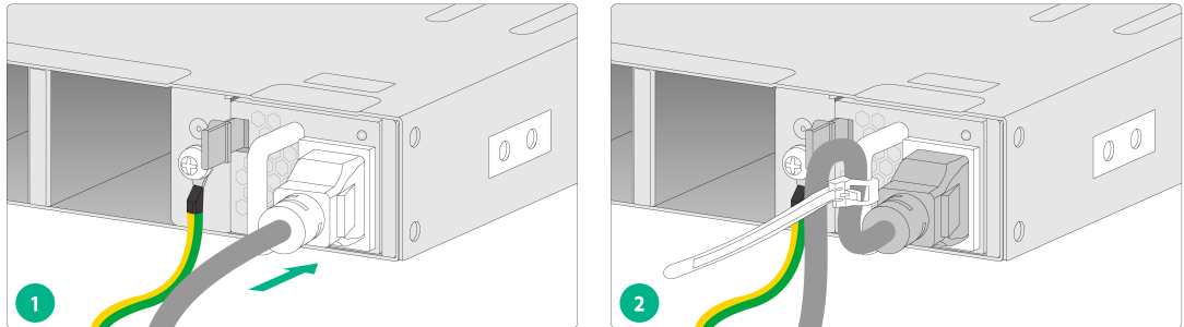
图2-23 连接交流电源线
