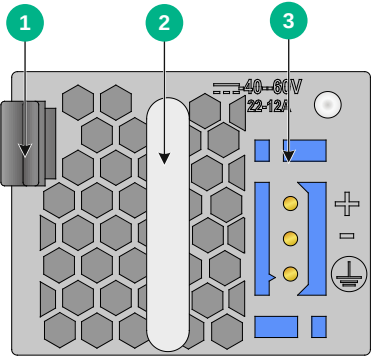
图A-4 PSR650B-12D1 直流电源模块外观
