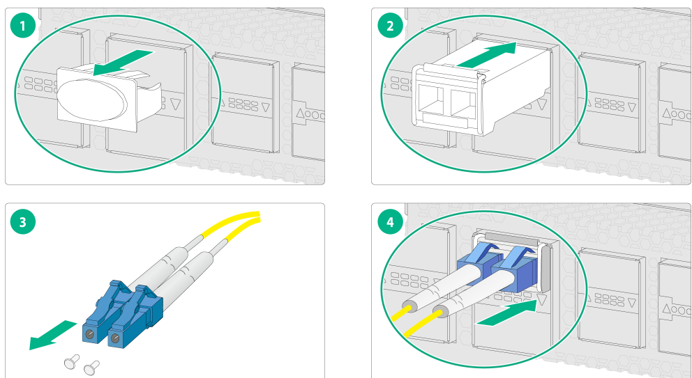
图2-21 安装光模块和光纤示意图（LC 型接口）
