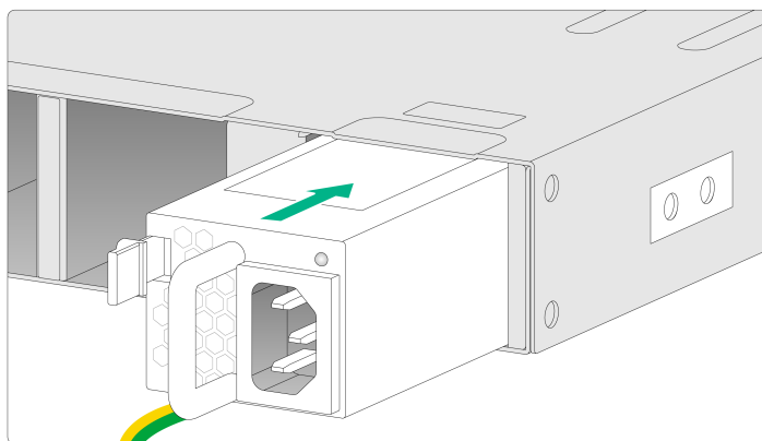
图2-12 安装交流电源模块
