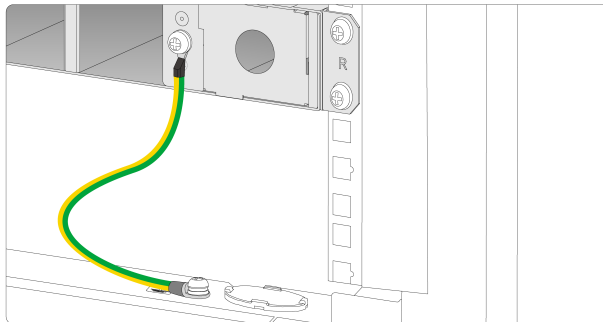
图2-9 连接到机柜接地
