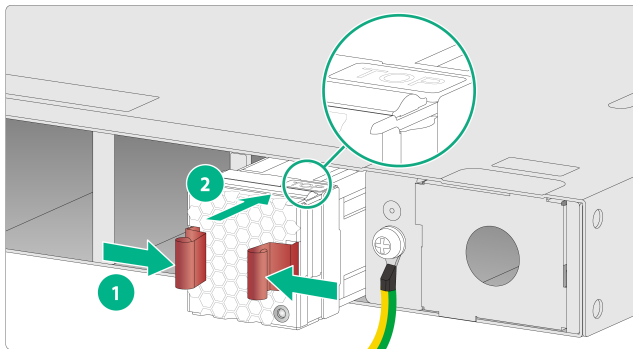
图2-10 安装风扇模块
