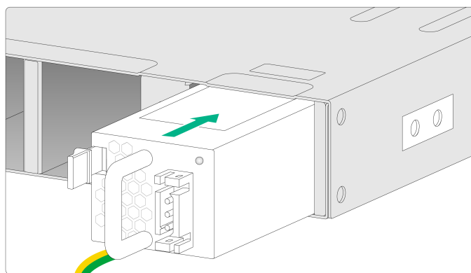
图2-13 安装直流电源模块
