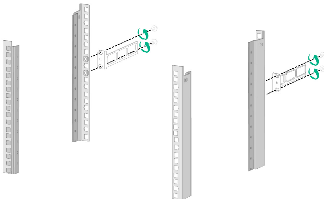
图2-5 安装后挂耳（后挂耳反装）
