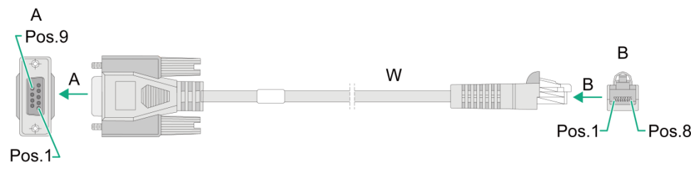
图C-1 CONSOLE 口和 PC 机（或终端）的串口之间电缆示意图。
