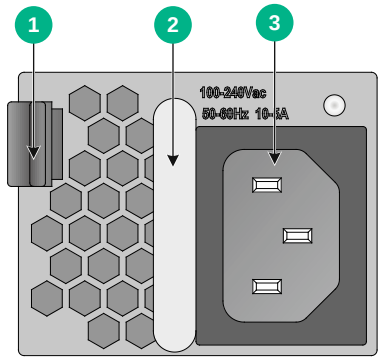
图A-3 PSR650B-12A1 交流电源模块外观
