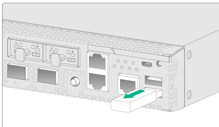
图4-3 更换 U 盘
